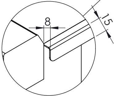
DETTAGLIO SCALA 1 : 2
